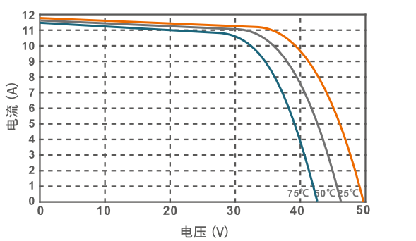
不同温度条件下的电压、电流曲线图
